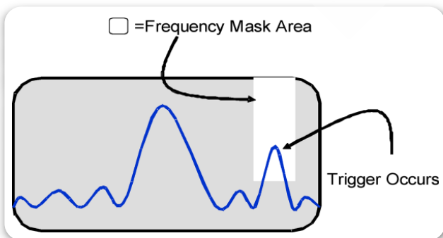
▶ 图 4-5. 采用频率模板的实时频域触发
