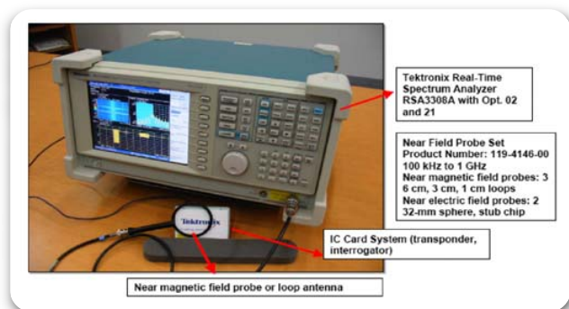
► 图 4-27. RFID 测试实物配置
