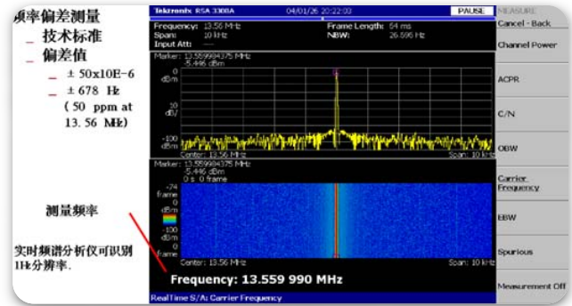
▶ 图 4-14. 通过“Carrier Frequency”键进行载波频率测量，在屏幕下端直观地显示测量结果
