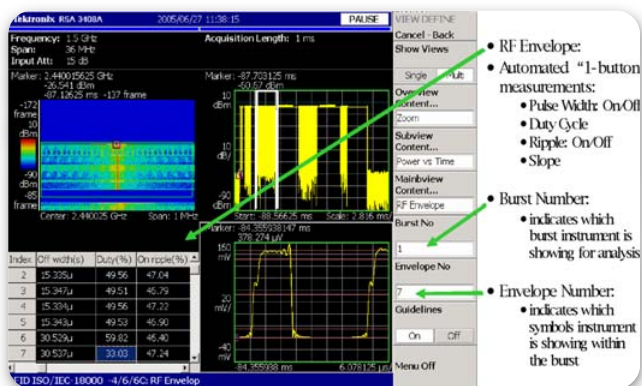
▶ 图 4-19. 通过“RF Envelop”键进行射频包络测量,如 RF 包络的开机和关机纹波、占空比和脉宽。
