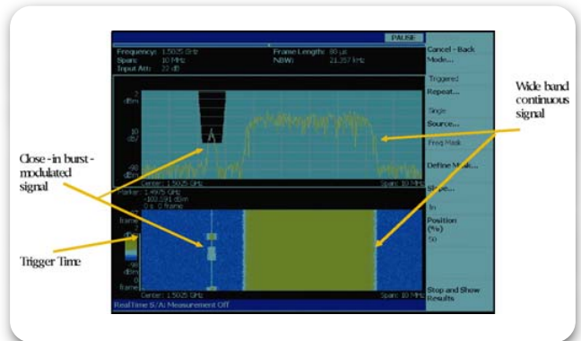
▶ 图 4-6. 使用频率模板，在存在大的信号时触发低电平脉冲。
