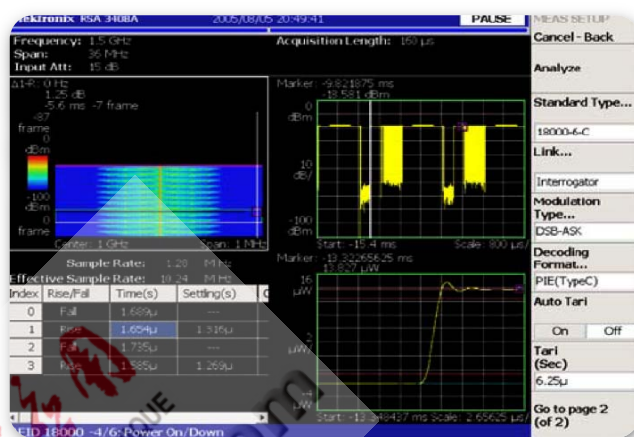
▶ 图 4-18. 在 RTSA 中,用户只需按一个键,就可以在查询会话中进行开机和关机测量,确定是否符合行业标准。
