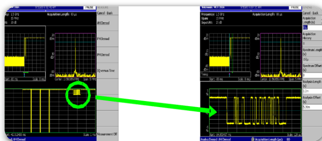
► 图 4-13. RTSA 捕获一段时间内的 RFID 信号并放大观察
