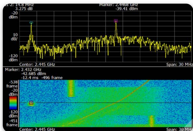
▶ 图4-17. 通过频域图和三维频谱图观察跳频信号(带有干扰信号)
