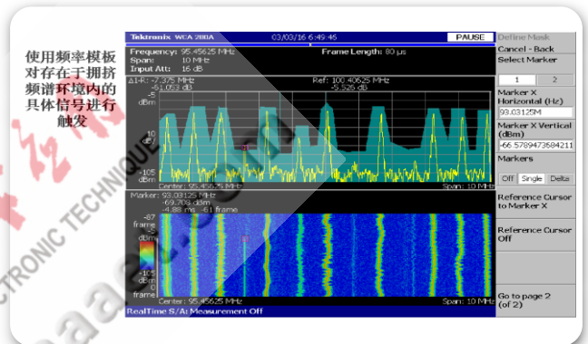
▶ 图 4-7. 使用频率模板，在拥挤的频谱环境中触发特定信号。
