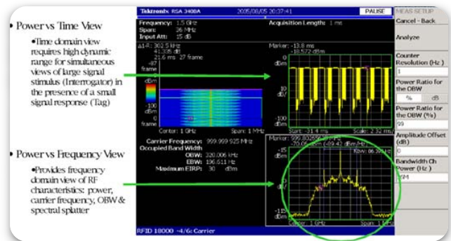
▶ 图 4-16. 通过通过显示频谱，进行 OBW/EBW 和 EIRP 测量
