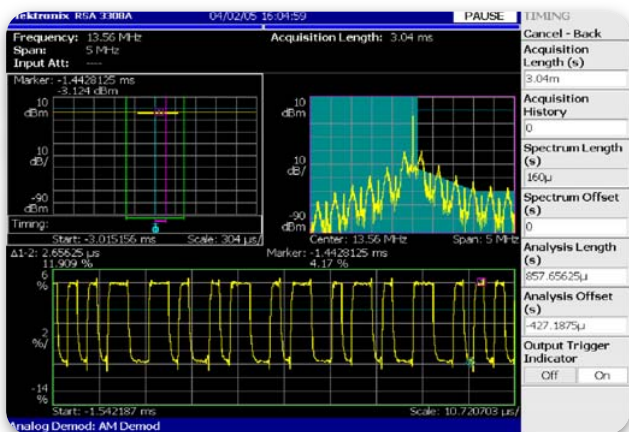
► 图 4-11. 显示功率随时间变化、功率与频率关系及 ASK 解调的多域图。
