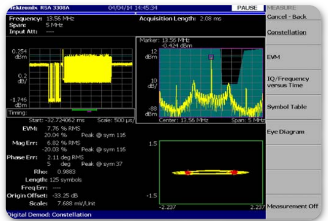
▶ 图 4-22. RTSA 对 RFID 信号解调，查看星座图和 EVM 等参数。
