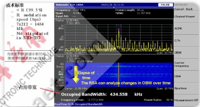
▶ 图 4-15. 通过“OBW”键进行占用带宽测量，在屏幕下端直观地显示测量结果
