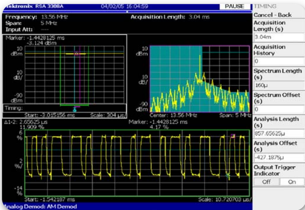
图 4-23. RTSA 对 RFID 的 ASK 调制信号解调, 分析 ASK 调制的时间序列。
