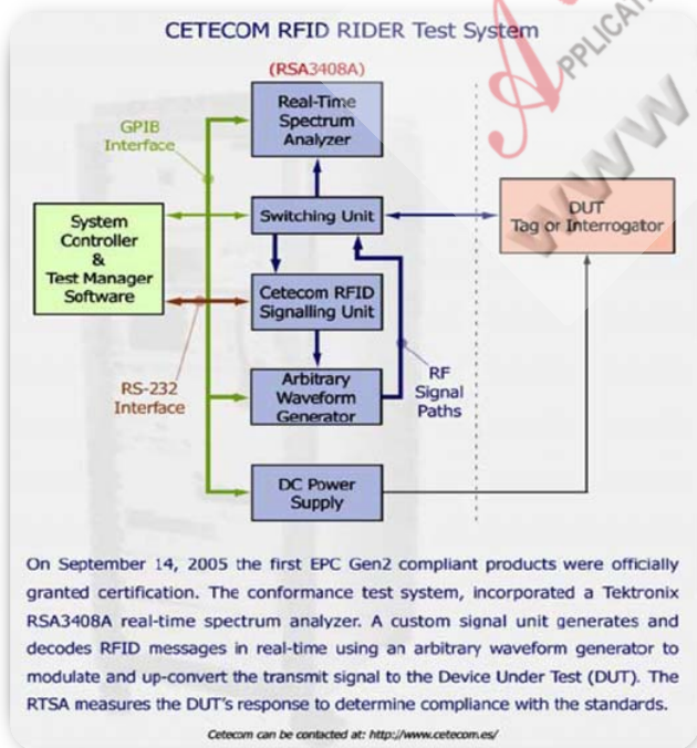
► 图 4-26. EPC Gen2 一致性综合测试系统
