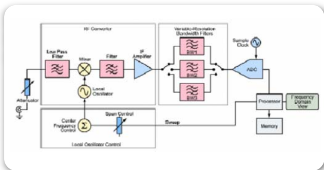
► 图 4-2. 典型的扫描式频谱分析仪结构图。
