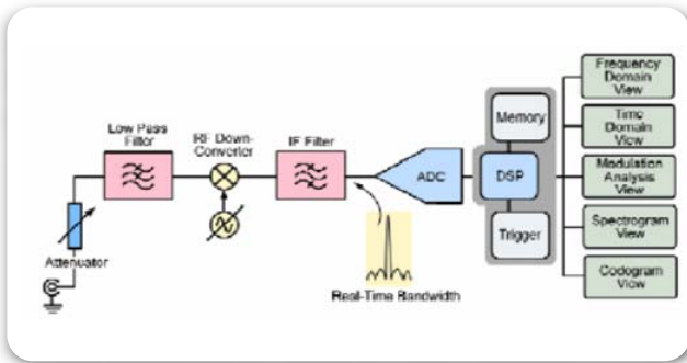
▶ 图 4-4. 实时频谱分析仪简化框图
