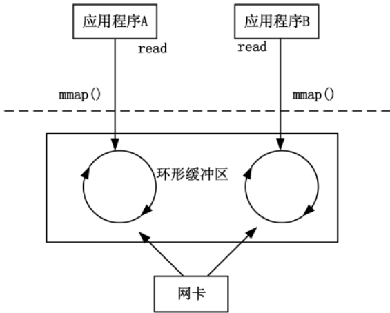
图 1 PF_RING 结构
