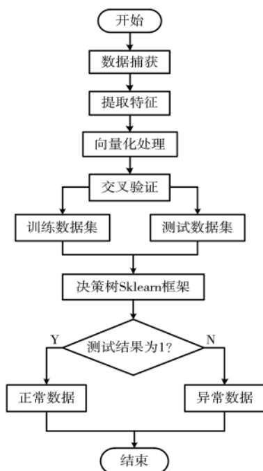
图 2 决策树算法分类模型构建流程图
