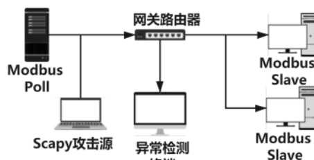
图 3 模拟通信拓扑图
