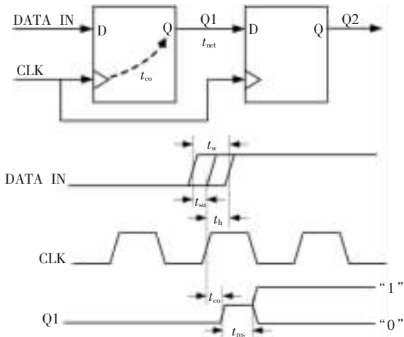
图1 亚稳态产生示意图
