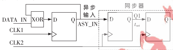
图 4 脉冲扩展同步电路
