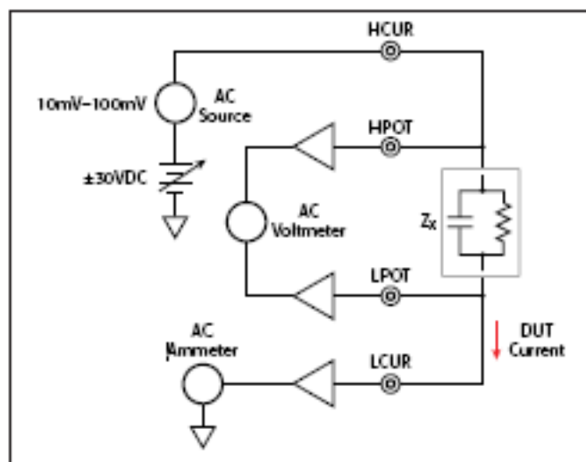
图3. C-V测量的基本测试配置
