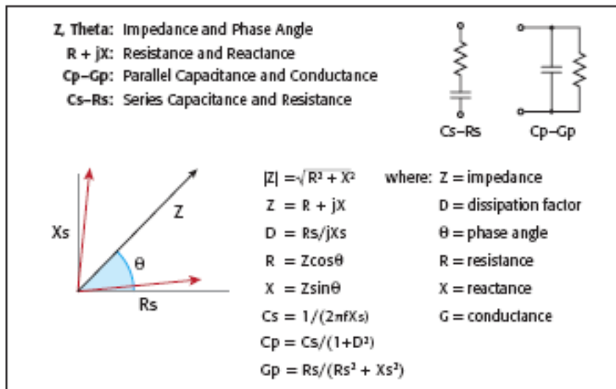
图4. C-V测量得到的主要电气变量
