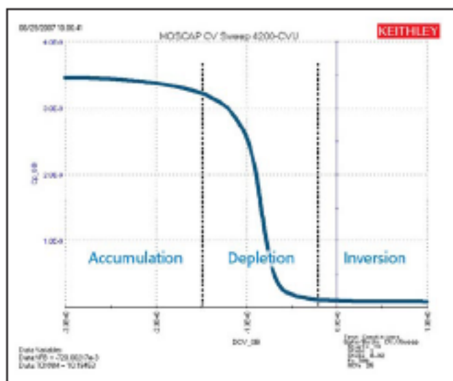
图2. C-V测试中获得的MOSCAP结构的直流偏压扫描
