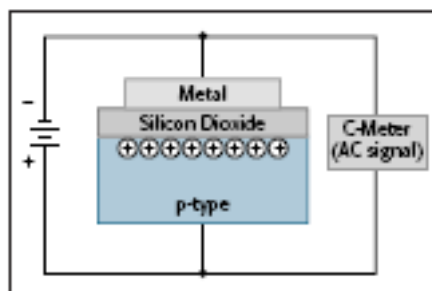
图1. P型衬底上形成的MOSCAP结构的C-V测量电路
